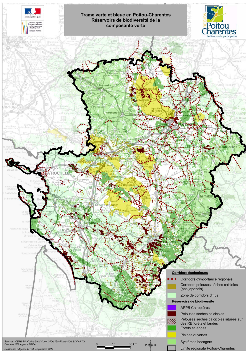
Figure 5. Cartographie de la composante verte
