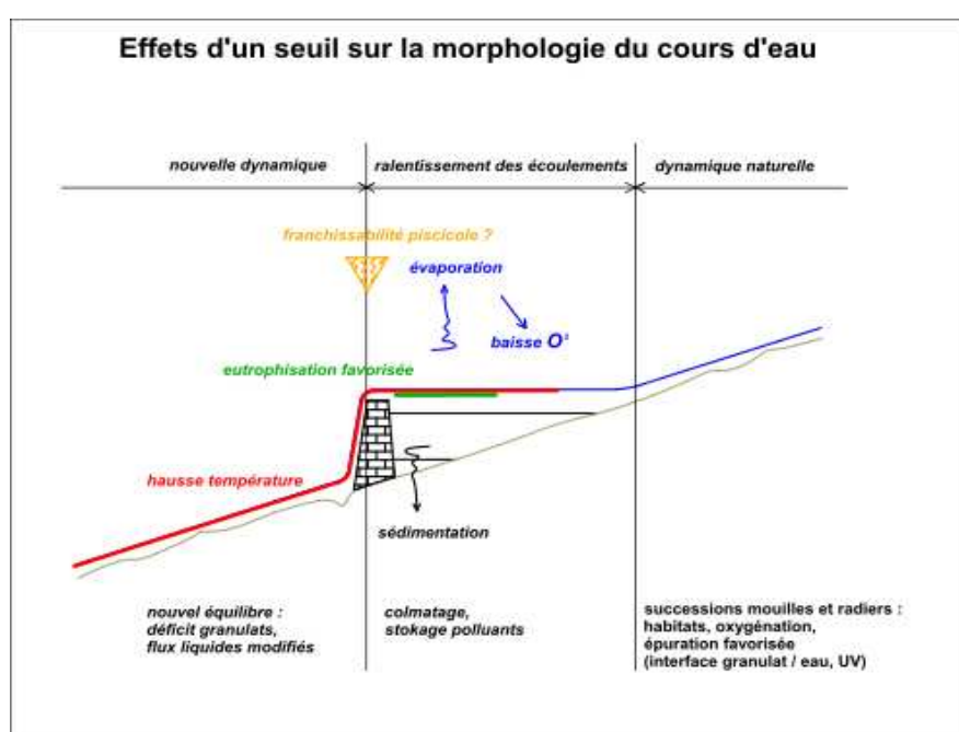
Figure 90. Effet d'un seuil sur la morphologie d'un cours d'eau (Sources : DREAL Poitou-Charentes)
